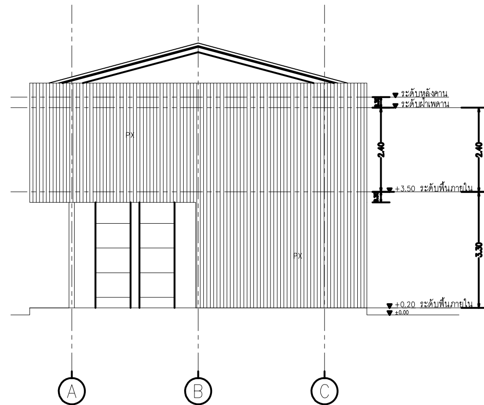
รูปด้าน ④ 1:100
