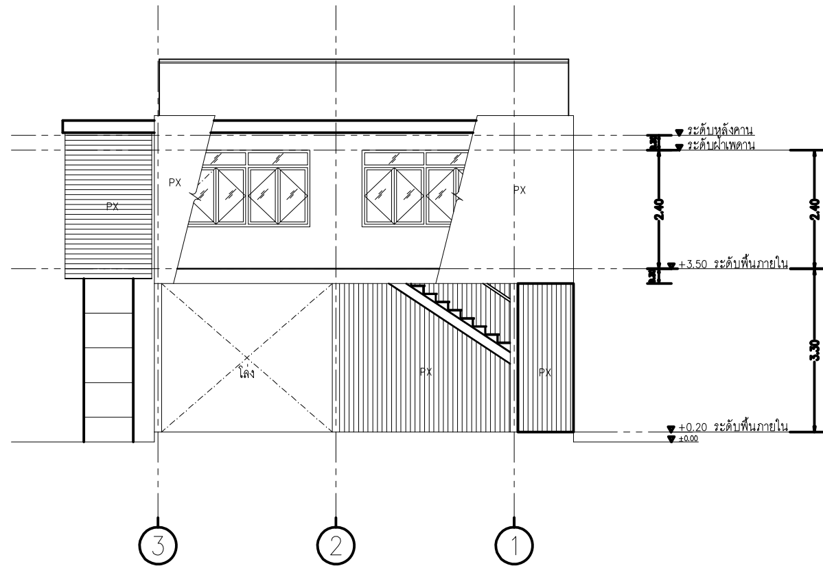
รูปด้าน ③ 1:100
