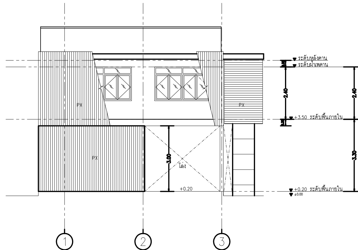
รูปด้าน ๑ 1:100
